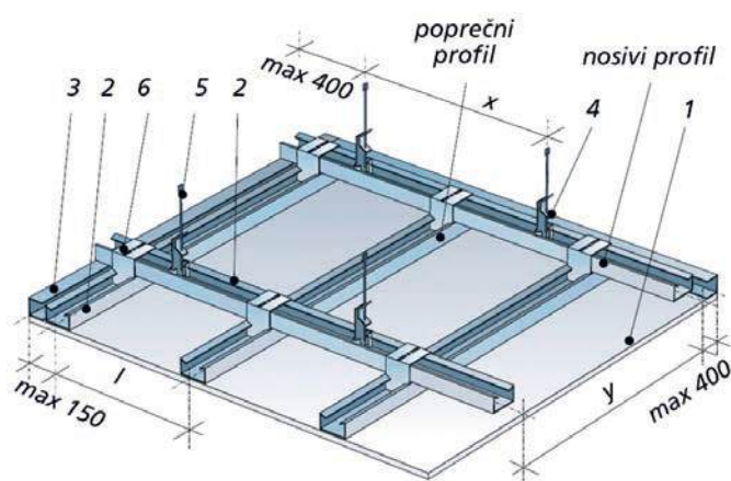
Slika 2-73 Metalna potkonstrukcija spušenog stropa u dva nivoa [99]
