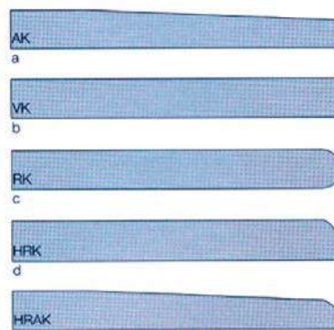
Slika 1-39 Različite izvedbe rubnih završetaka gipskartonskih ploča [38]
