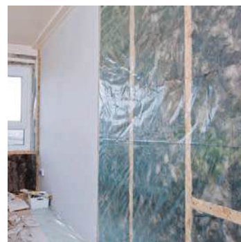
Slika 2-13 Prikaz postavljanja toplinske izolacije od mineralne vune te postavljanje parne brane na drvenu potkonstrukciju [93], [94]
