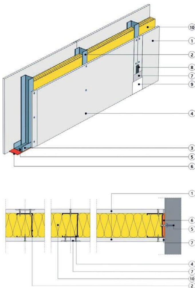
Slika 2-49 Pregradni zid s jednostrukom metalnom potkonstrukcijom [99]
