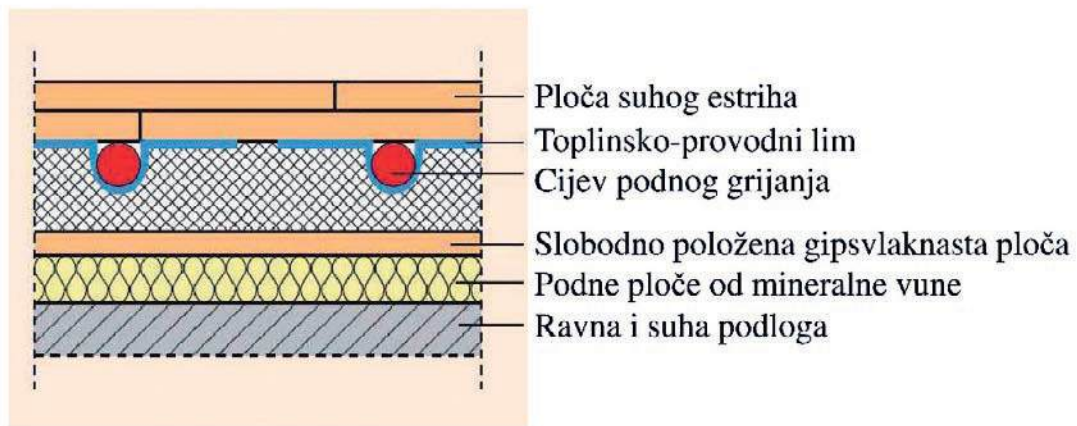
Slika 2-135 Primjer sustava podnog grijanja na dodatnu izolacijsku ploču od mineralne vune sa slobodno postavljenom gipsvlaknastom pločom [180]
