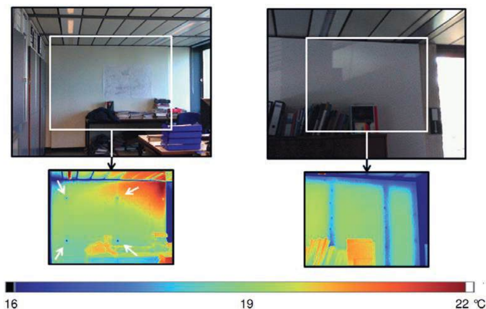
Slika 2-41 Toplinski mostovi uzrokovani metalnim pričvrsnicama, odnosno metalnim nosačima potkonstrukcije [98]
