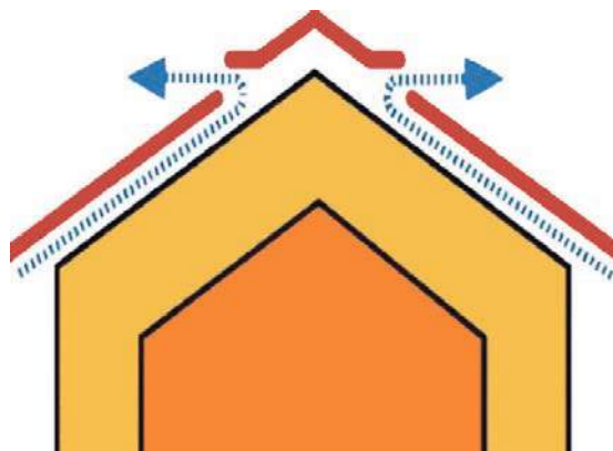
Slika 2-95 Strujanje zraka od okapnice do izlaza na sljemeni [132]
