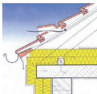
Hladni krov
