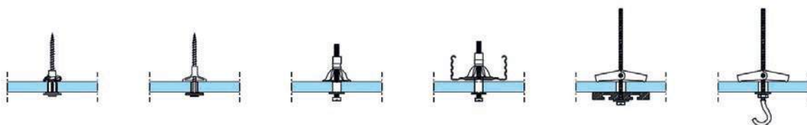
Slika 2-86 Ovjes tereta na spuštene strop [91]
