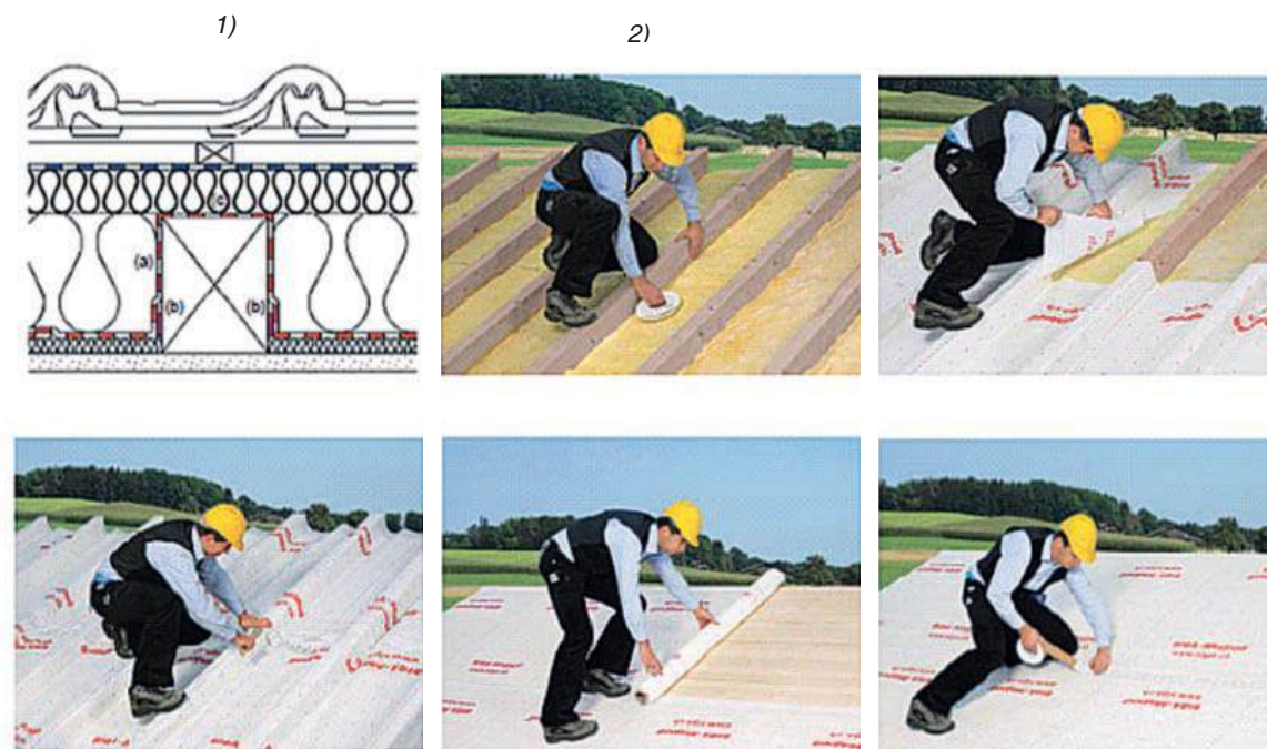
1) poprečni presjek ventiliranog krova 2) pažljivi rad na polaganju i zatvaranju spojeva parne brane
