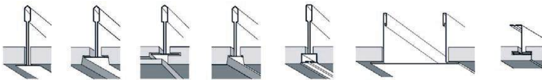
Slika 2-67 Ovjesni sistemi spušenog stropa s vidljivom potkonstrukcijom [124]
