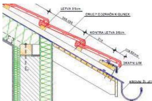
Drvena konstrukcija
